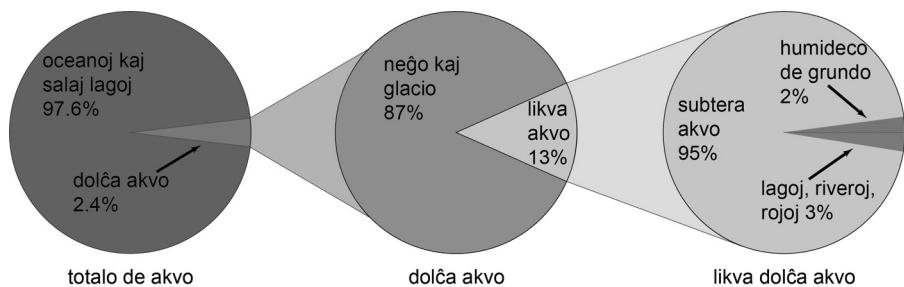
Bildo 1: Distribuo de akvo sur la planedo Tero.
